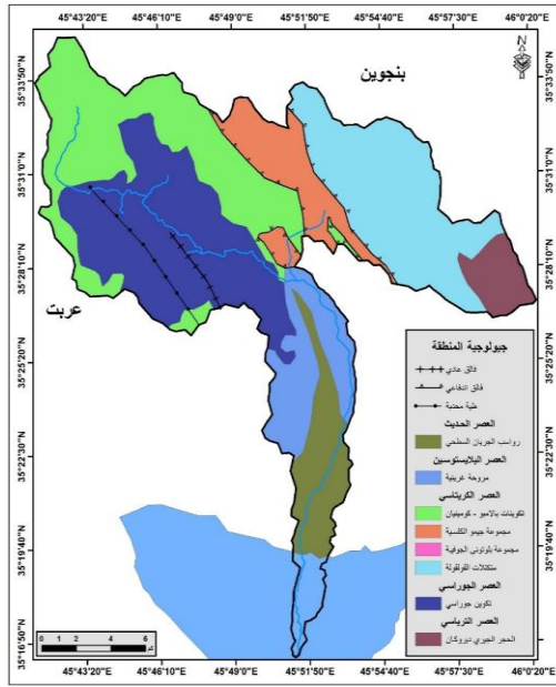
(خريطة 6) جيولوجية منطقة البحث
